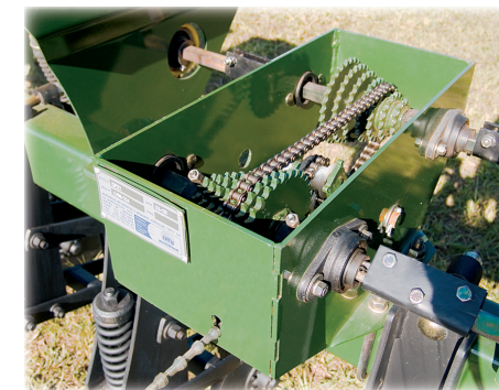
Varias regulaciones pueden ser rápidamente obtenidas a través de simple cambio de engranajes.
